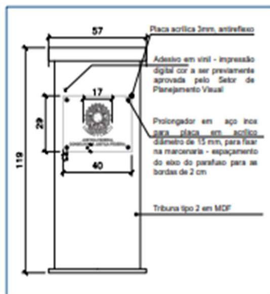
VISTA FRONTAL - PLACA P/ TRIBUNA TIPO 2
